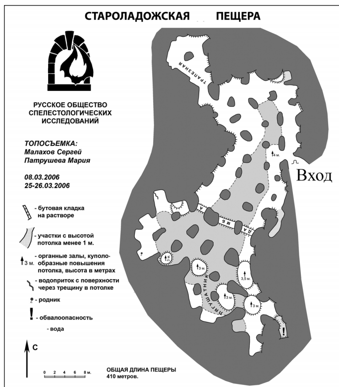
План Староладожской подземной выработки. Топо съемка С. Малахов, М. Патрушева. 2006 год
