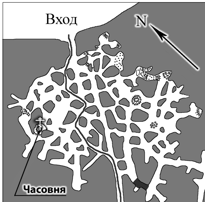
Фрагмент плана подземной выработки «Береговая» в Саблино. Топо съемка по материалам Ю.С. Ляхницкого
